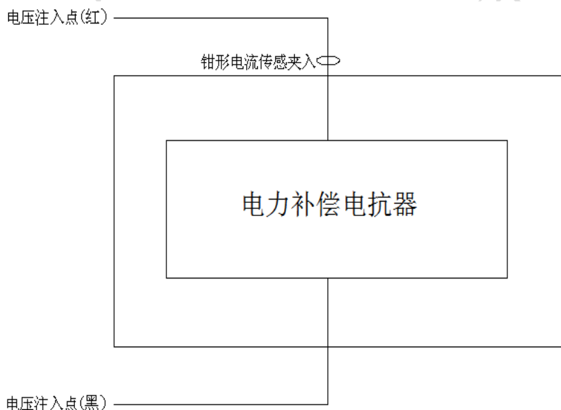
被试电抗器电感接线图
