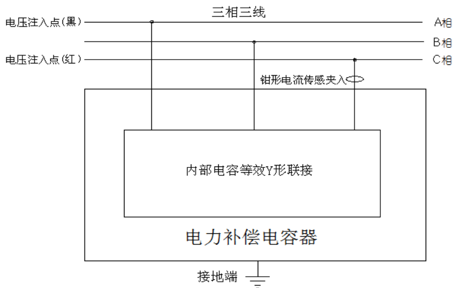
Y 形联接被试电容 CA 相接线图
