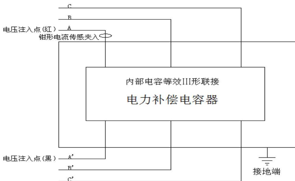
III形联接被试电容接线图
