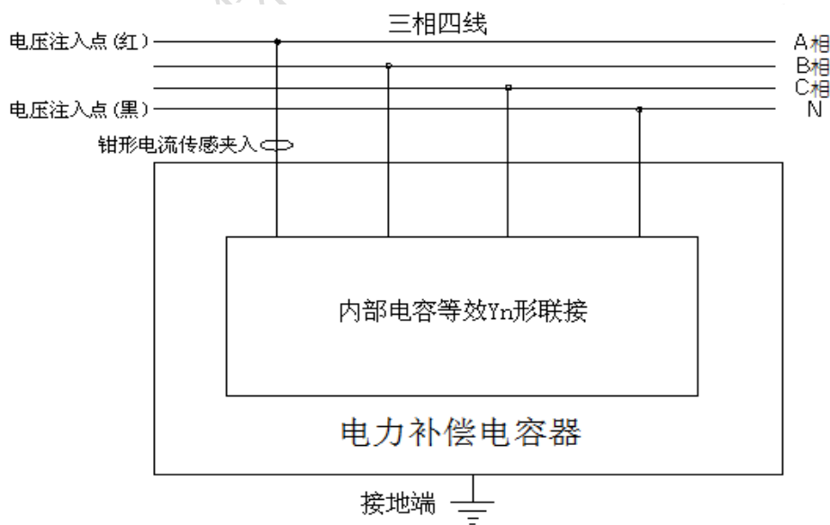
Yn 形联接被试电容 An 相接线图
