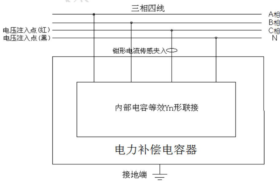
Yn 形联接被试电容 Cn 相接线图
