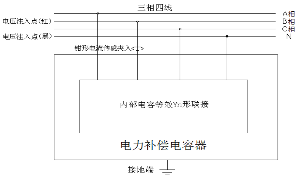
Yn 形联接被试电容 Bn 相接线图
